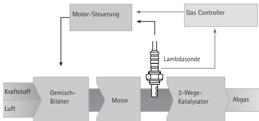
Funktionsweise der Lambdasonde
